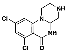
7,9-Dichloro-1,2,3,4,4a,5-hexahydropyrazino[1,2-a]quinazolin-6-one
