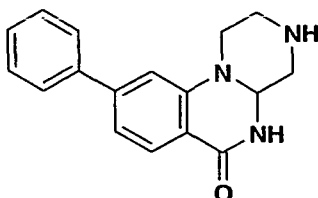
9-Phenyl-1,2,3,4,4a,5-hexahydropyrazino[1,2-a]quinazolin-6-one
