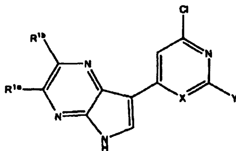
formule (I)
