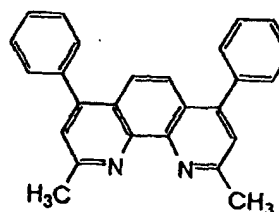
BCP
