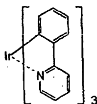
Ir(ppy) 3
