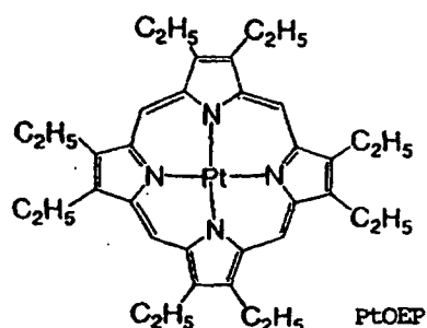
PtOEP
