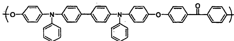
TPDPEK
