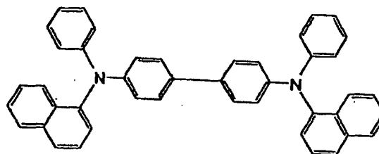
\alpha -NPD
