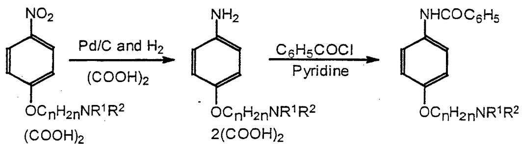
SCHEME 3 (method E):
