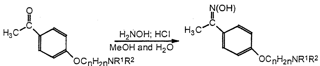
SCHEME 5 (method J):
