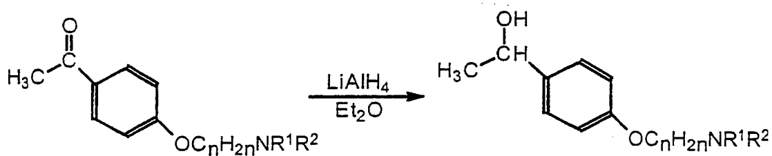
SCHEME 4 (method G):
