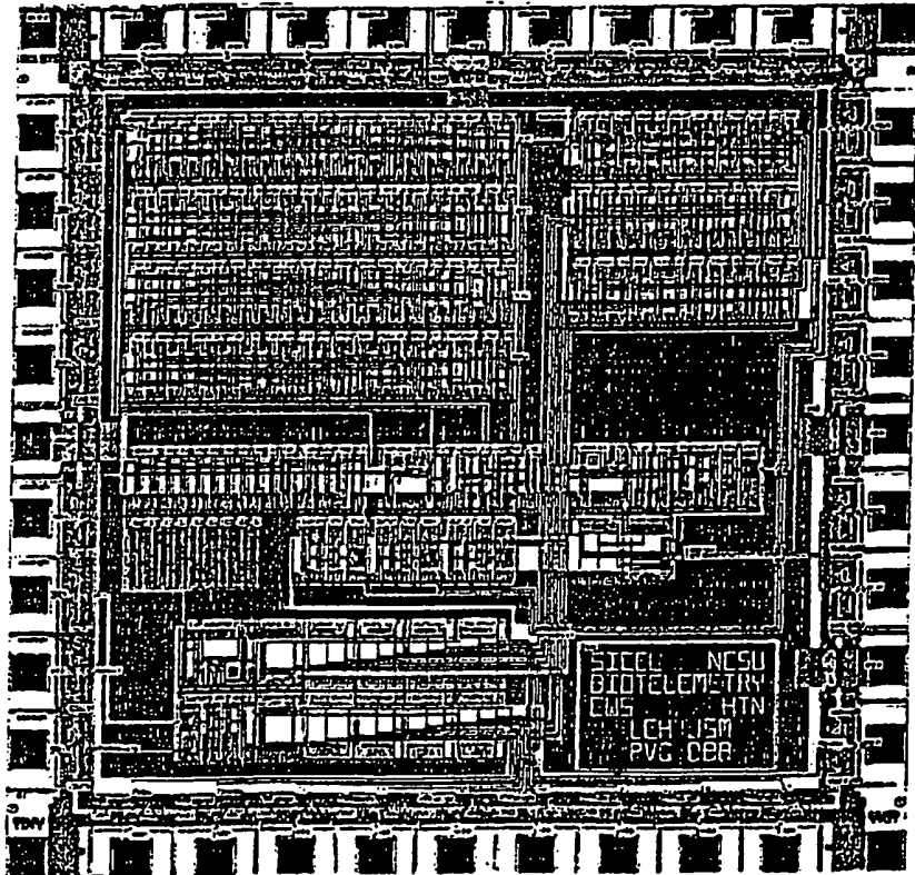
IC LAYOUT
