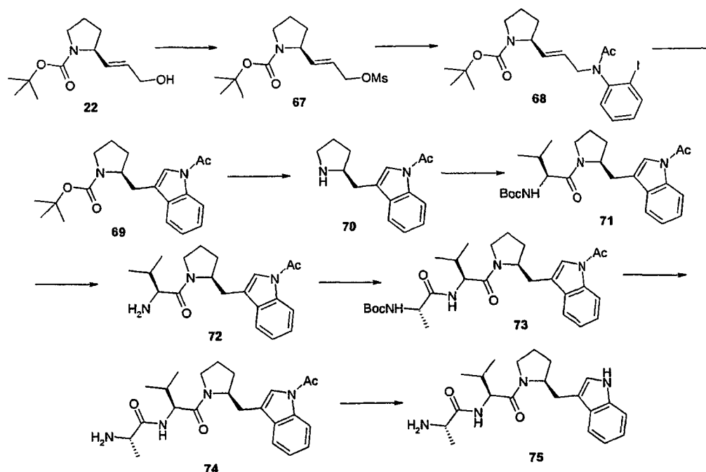
Scheme VI
