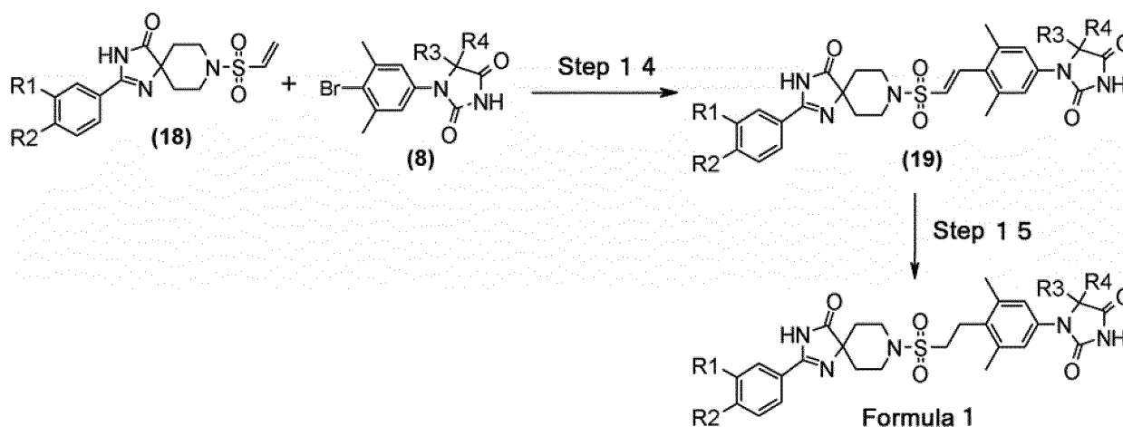
Scheme 6 (Method B)
