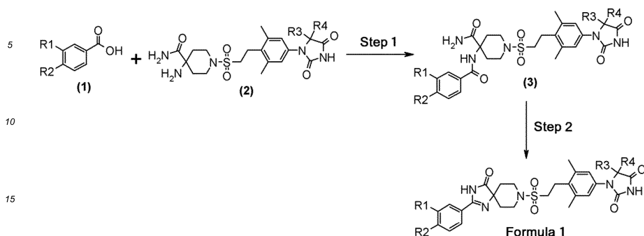
Scheme 1 (Method A)
