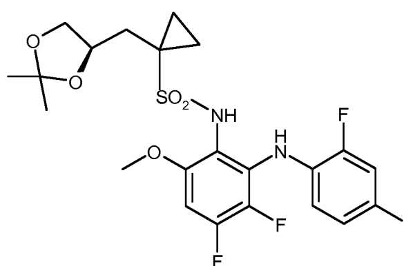
55 ((R)-13)
