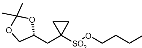
(R)-6 ;
