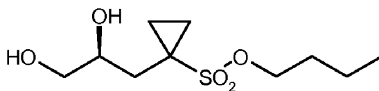
(S)-5 ;
