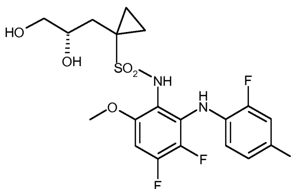
55 (S)-14 ;
