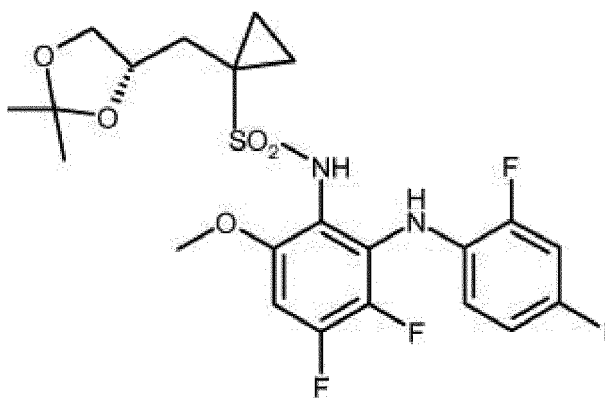
((S)-13);
