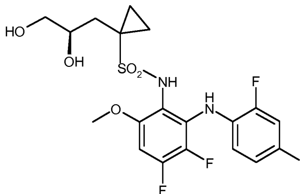
(R)-14 ;
