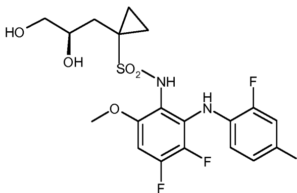
55 ((R)-14 ;
