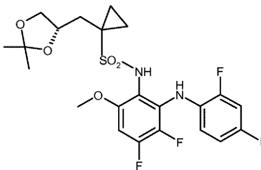
((S)-13);
