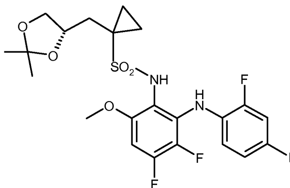
((S)-13)
