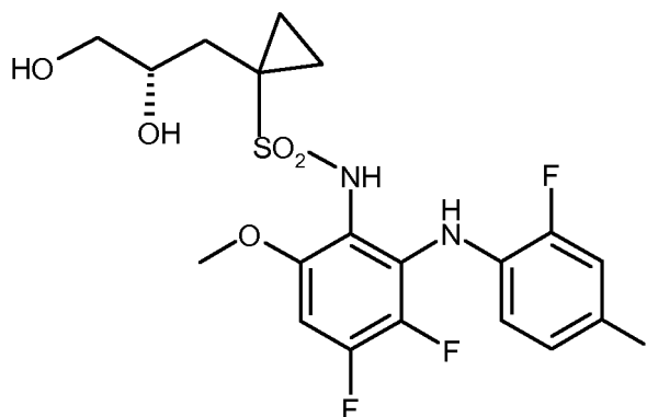
(S)-14 ;
