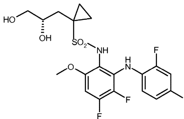
(S)-14 ;
