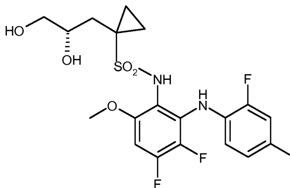
(S)-14 ;
