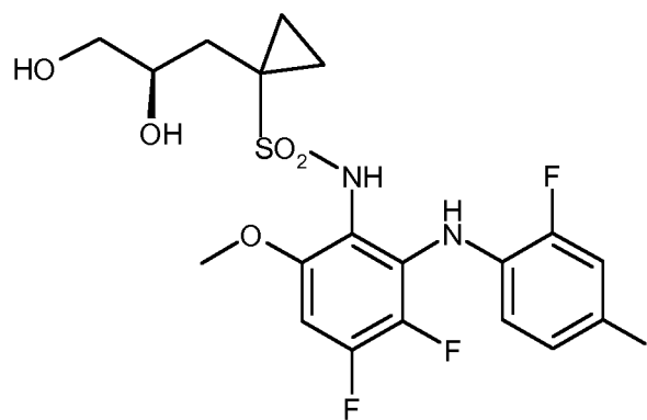
15 (R)-14 ;
