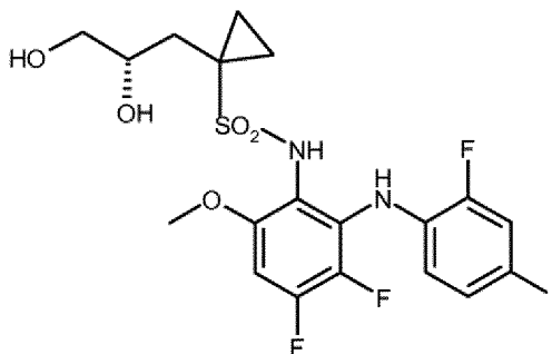
(S)-14 ;
