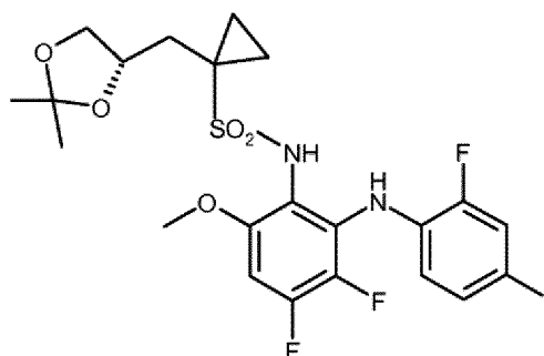
((S)-13)
