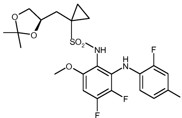
35 ((R)-13) ;
