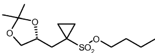
(R)-6 ;
