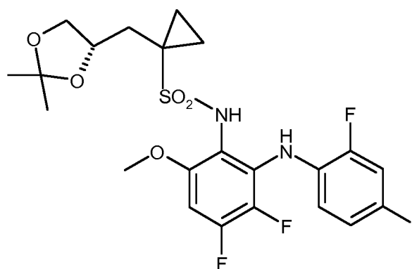
((S)-13)
