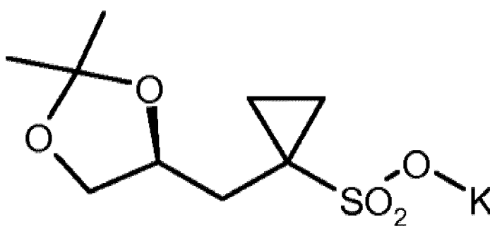
(S)-7';
