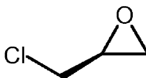
(S)-1 ;
