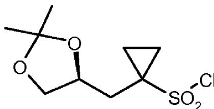
(S)-10 ;
