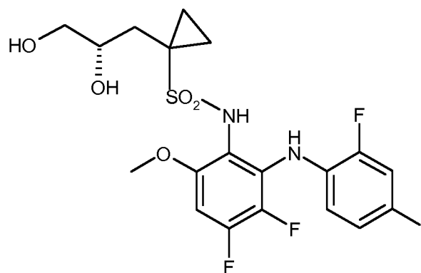
(S)-14 ;
