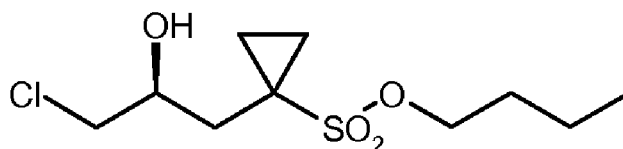
(S)-3 ;
