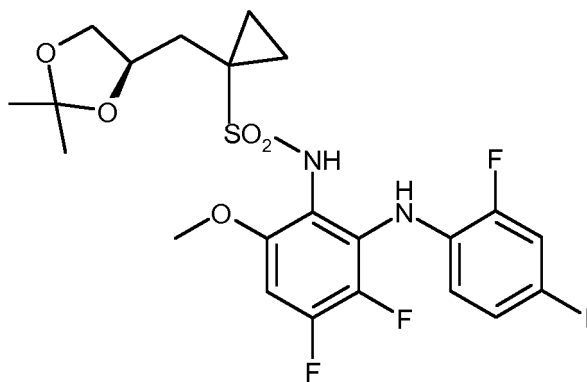
((R)-13)
