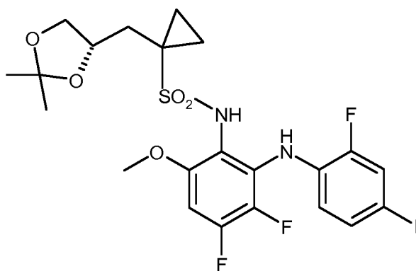
((S)-13)
