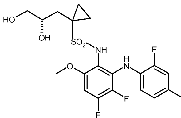
15 (S)-14 ;
