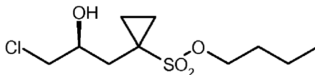
(S)-3 ;
