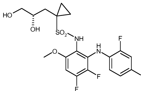
15 (S)-14 ;
