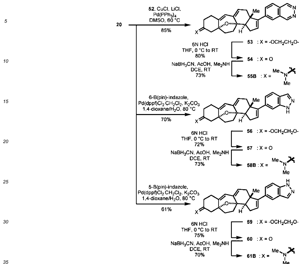
Scheme 3-4.
