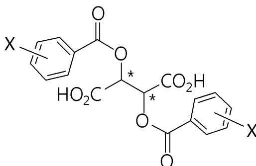
[Formule Chimique 1]
