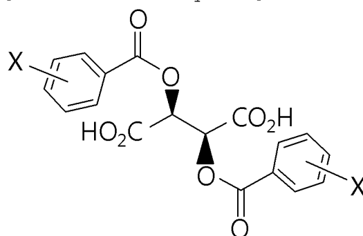
[Formule Chimique 2]
