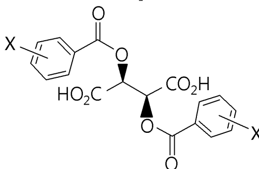
[Formule Chimique 2]
