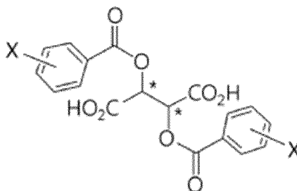
[Chemische Formel 1]
