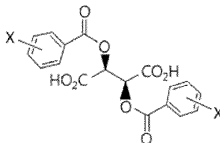
[Chemische Formel 2]
