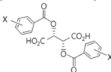
[Chemische Formel 3]
