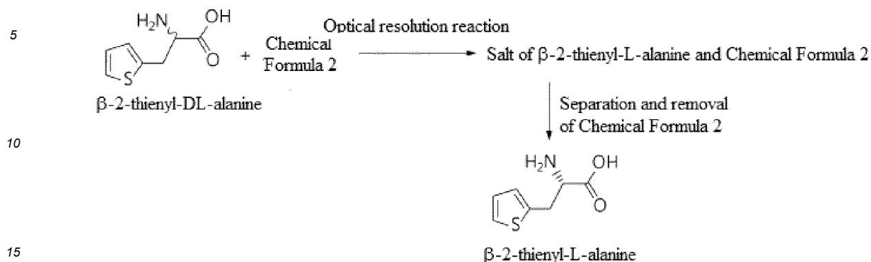
[Scheme 1]
