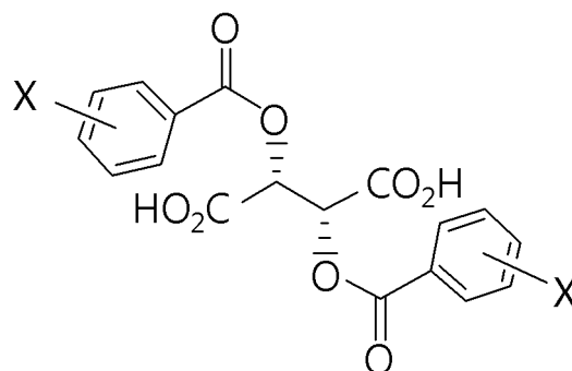
[Formule Chimique 3]
