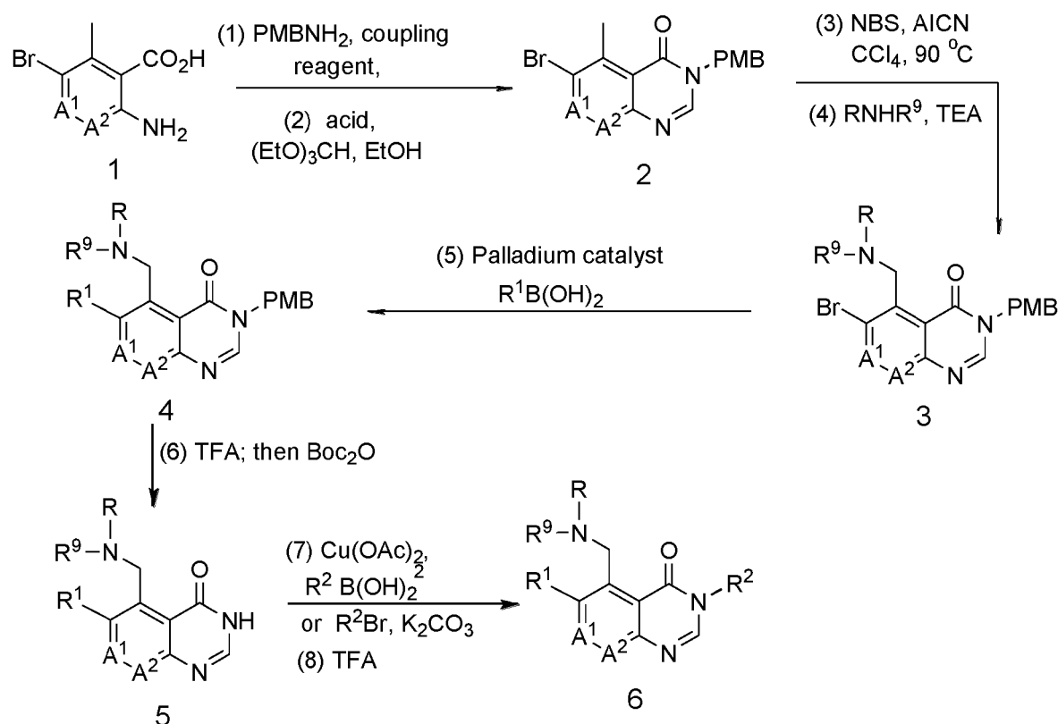
Scheme A:
