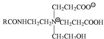
(DI)PROPIONATE
