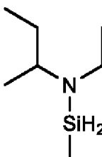
N-sec-butyl-N-éthylamino-méthylsilane,
