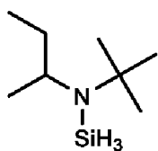
N-sec-butyl-N-tert-butylaminosilane,
