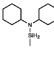
N,N-dicyclohexylamino-méthylsilane,
