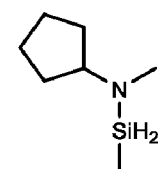
N-méthyl-N-cyclopentylamino-méthylsilane,
