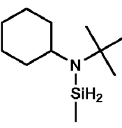
N-tert-butyl-N-cyclohexylamino-méthylsilane,
