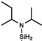
N-sec-butyl-N-iso-o-propylamino-méthylsilane,
