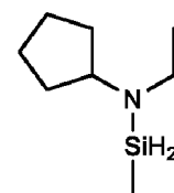
N-méthyl-N-cyclopentylamino-méthylsilane,
