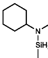
N-cyclohexyl-N-méthylamino-méthylsilane,
