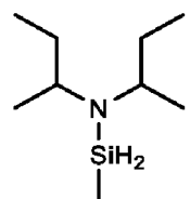
N,N-di-sec-butylamino-méthylsilane,
