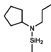
N-cyclopentyl-N-n-propylamino-méthylsilane,
