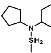
N-sec-butyl-N-cyclopentylamino-méthylsilane,
