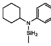
N-cyclohexyl-N-phénylamino-méthylsilane,
