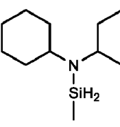
N-sec-butyl-N-cyclohexylamino-méthylsilane,
