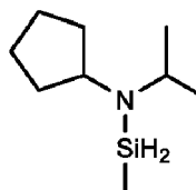
N-cyclopentyl-N-iso-propylamino-méthylsilane,
