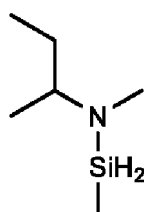
N-sec-butyl-N-méthylamino-méthylsilane,
