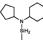
N-cyclohexyl-N-cyclopentylamino-méthylsilane,
