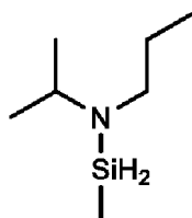
N-n-propyl-N-iso-propylamino-méthylsilane,
