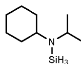
N-cyclohexyl-N-isopropylaminosilane
