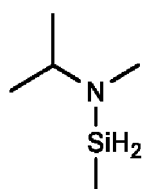
N-méthyl-N-iso-propylamino-méthylsilane,
