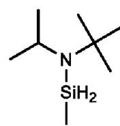
N-tert-butyl-N-iso-propylamino-méthylsilane,
