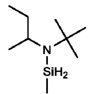
N-sec-butyl-N-tert-butylamino-méthylsilane,
