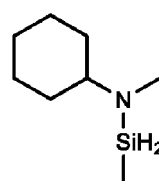
N-cyclohexyl-N-méthylamino-méthylsilane,
