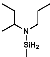
N-sec-butyl-N-n-propylamino-méthylsilane,
