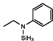
N-éthyl-N-phenylaminosilane,
