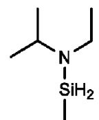
N-éthyl-N-iso-propylamino-méthylsilane,
