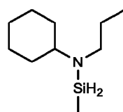
N-cyclohexyl-N-n-propylamino-méthylsilane,
