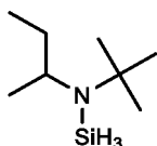
N-sec-butyl-N-tert-butylaminosilane,
