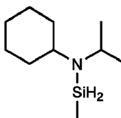
N-cyclohexyl-N-iso-propylamino-méthylsilane,
