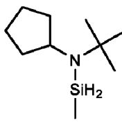
N-tert-butyl-N-cyclopentylamino-méthylsilane,
