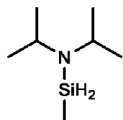
N,N-di-iso-propylamino-méthylsilane,
