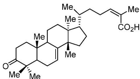
24-Z-masticadienonic acid (MDA)
