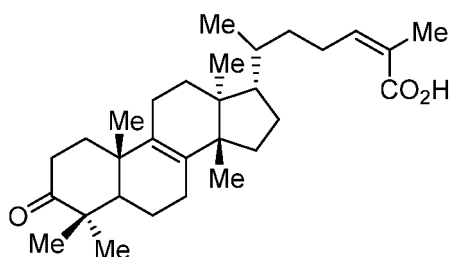
24-Z-isomasticadienonic acid (IMDA)
