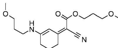
3-ethoxypropyl (2Z)-cyano{3-[(3-methoxypropyl)amino]cyclohex-2-en-1-ylidene}ethanoate
