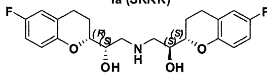
Ib (RSSS)
