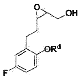
VI' (2R*,3S*)
