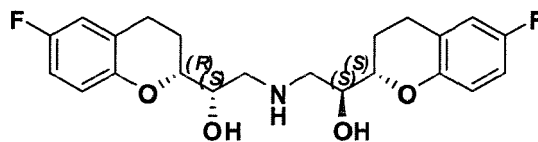
Ib (RSSS)
