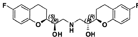
Ia (SRRR)
