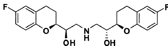
I (S*R*R*R*)
