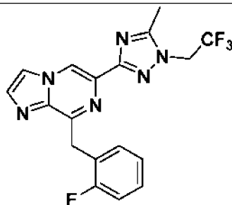
I-38
