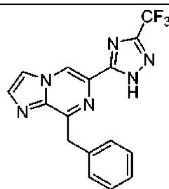
I-6
