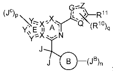
Formule IIB.
