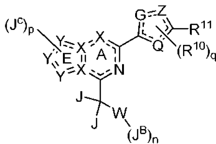
Formule I
