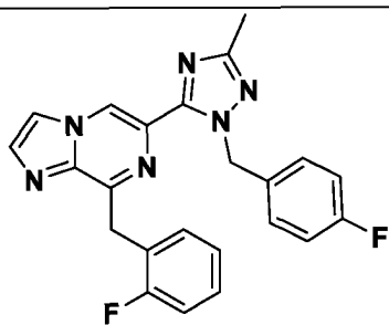
I-42
