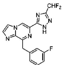
I-3
