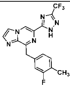
I-27
