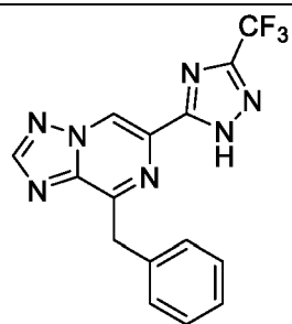
I-15
