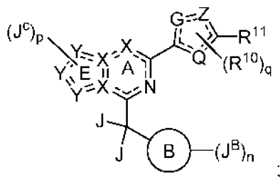
Formel IIB.
