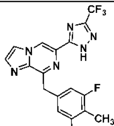
I-34
