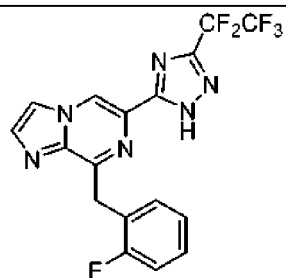
I-5
