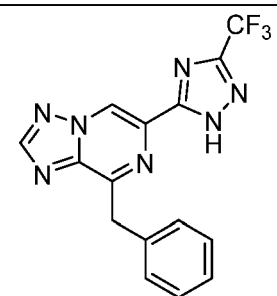
I-15
