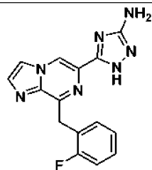
I-57
