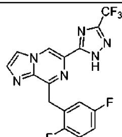
I-8
