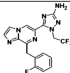
I-60
