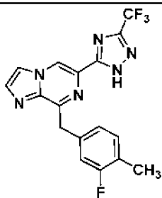
I-27
