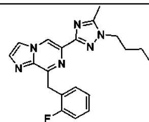
I-56
