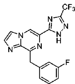
I-2
