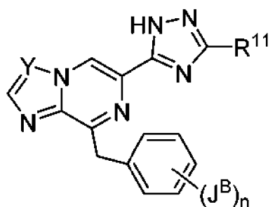
Formule V
