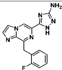
I-57
