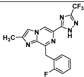
I-31
