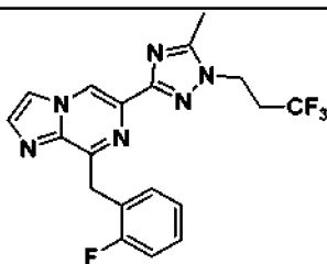
I-54
