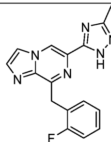
I-4
