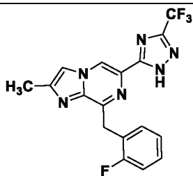
I-31
