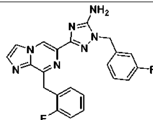
I-58
