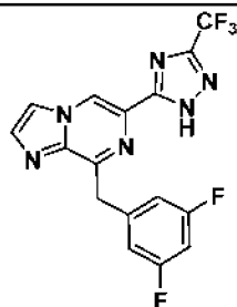
I-29
