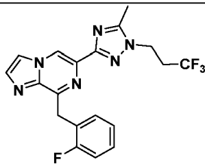
I-54
