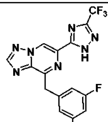
I-22
