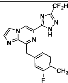
I-28
