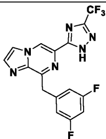
I-29
