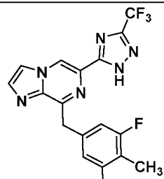
I-34
