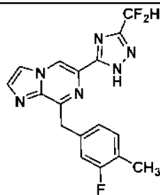
I-28
