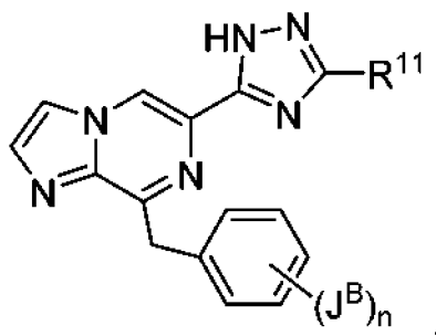
Formule VI
