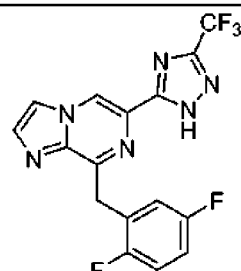
I-8
