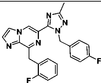
I-42
