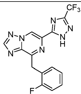
I-16
