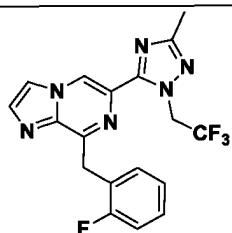
I-39
