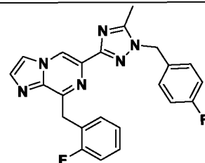
I-41
