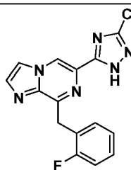
I-62
