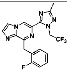
I-39
