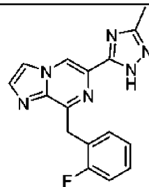
I-4
