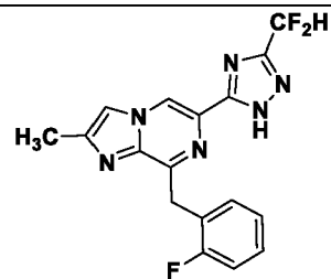
I-32
