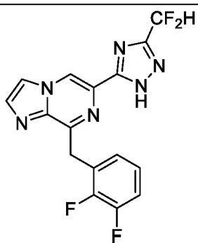
I-11
