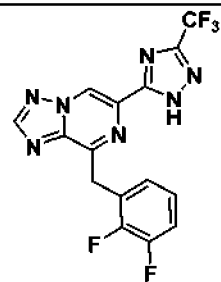
I-18
