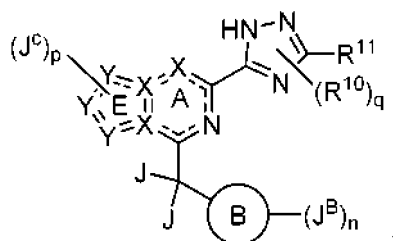
Formule III.
