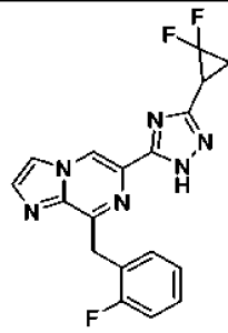
I-64
