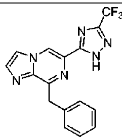
I-6
