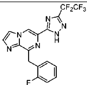
I-5
