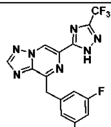
I-24
