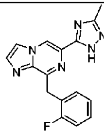
I-4
