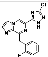
I-62
