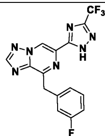
I-22
