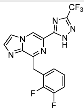
I-10
