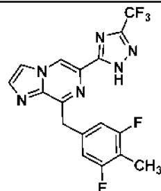
I-34
