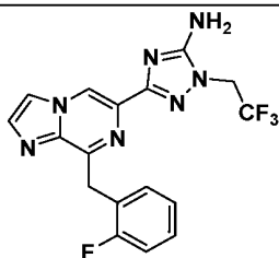
I-59
