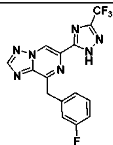
I-22
