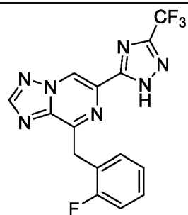
I-16
