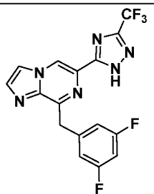
I-29
