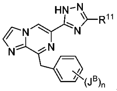
Formel VI
