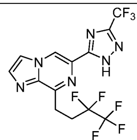
I-13
