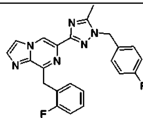
I-41
