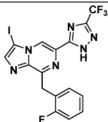
I-66
