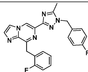
I-41
