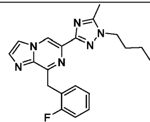
I-56
