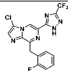
I-67
