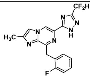
I-32
