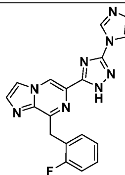
I-63
