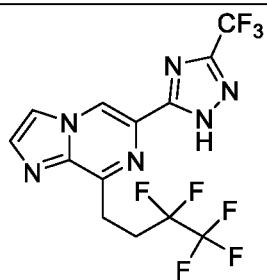
I-13
