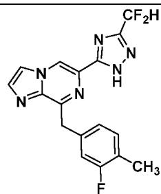
I-28
