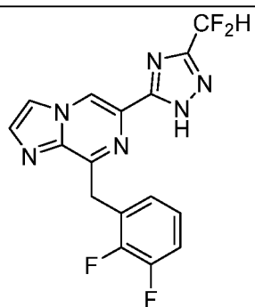
I-11
