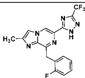
I-31
