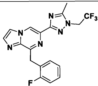
I-38
