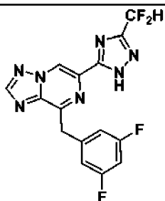
I-25
