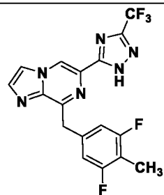
I-34
