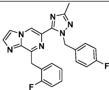
I-42
