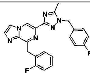
I-41
