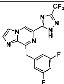
I-29
