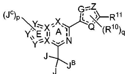
Formule IIA
