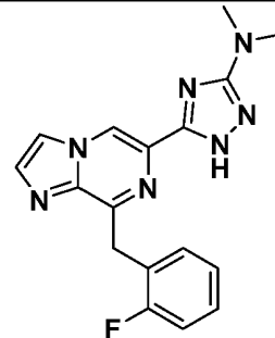
I-65
