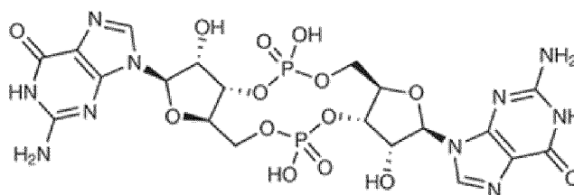
c-di-GMP
