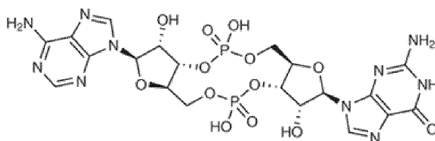
cGAMP (III)
