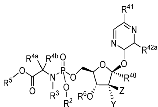
Formula VIId
