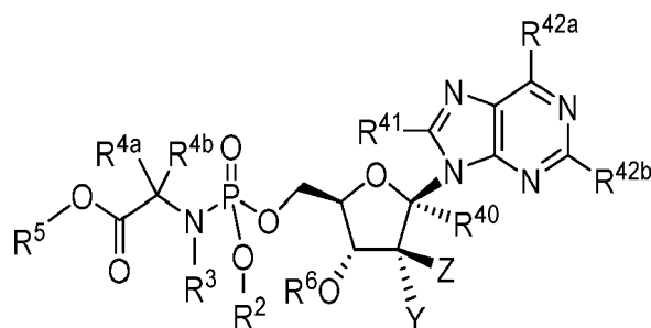
Formula VIIb
