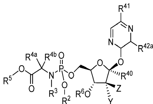
Formula VIId
