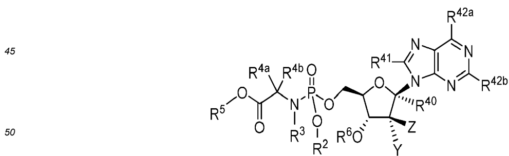
Formula VIIb
