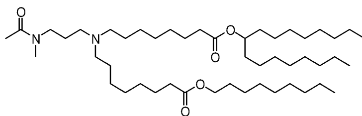
(Composé 196),
