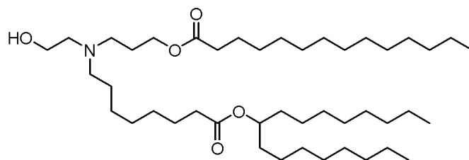
(Composé 97),
