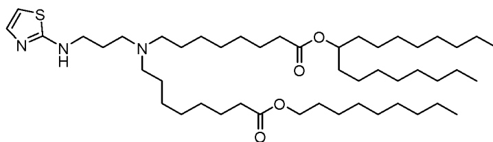
(Verbindung 208),
