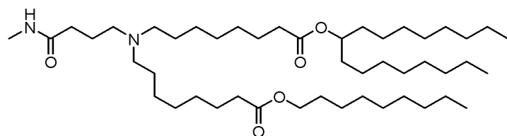
(Verbindung 223),
