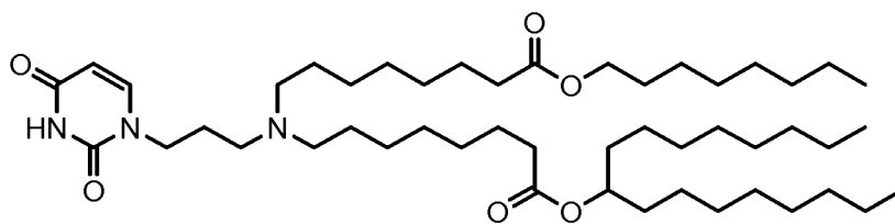
(Verbindung 43),
