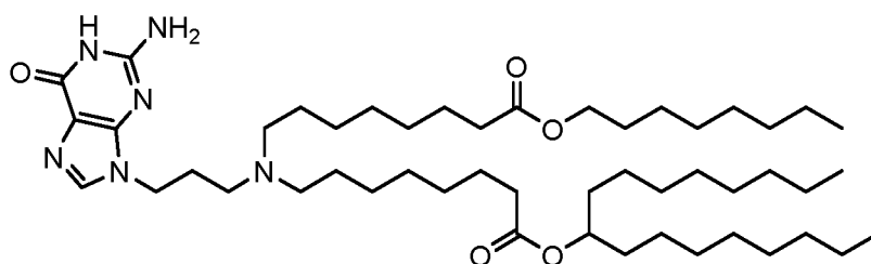
(Verbindung 46),
