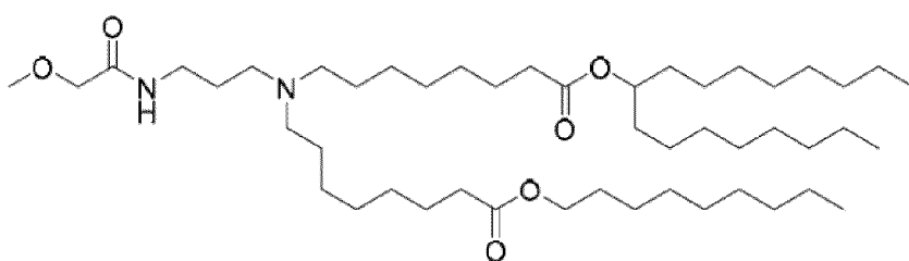
(Verbindung 178),
