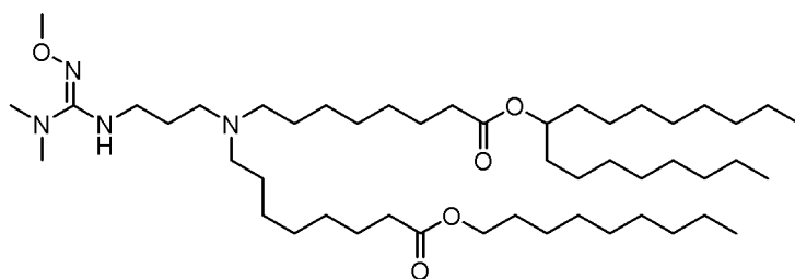
(Verbindung 211),
