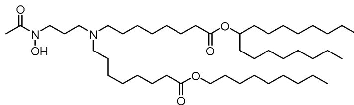
(Composé 204),
