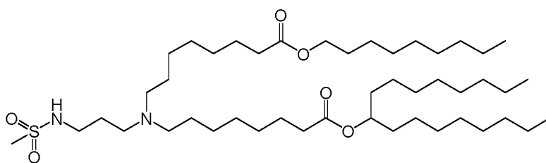
(Composé 109),
