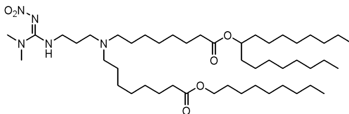
(Composé 209),
