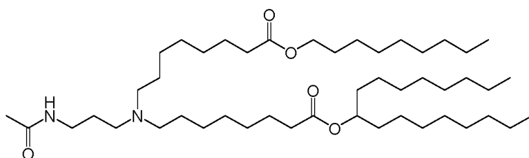
(Verbindung 108),
