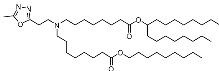
(Composé 231) ,
