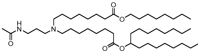
(Verbindung 37),
