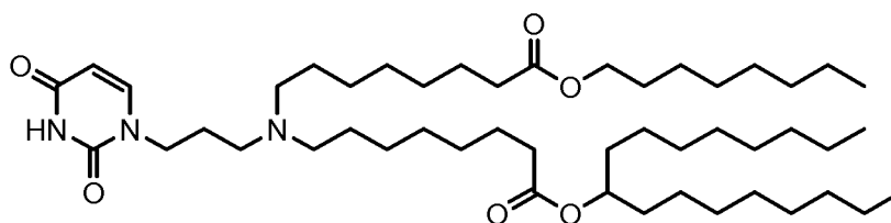
(Composé 43),
