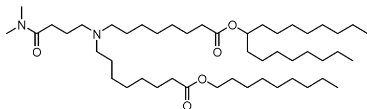
(Verbindung 224),
