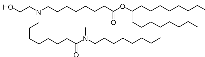
(Composé 145),
