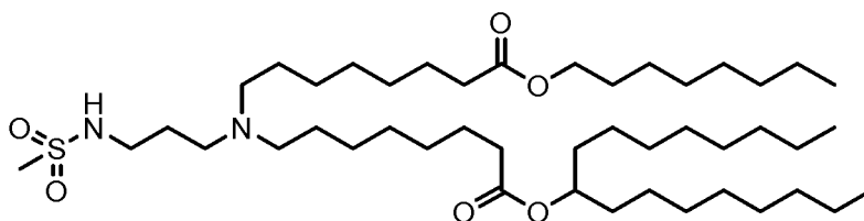
(Verbindung 38),
