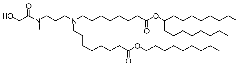
(Composé 198),
