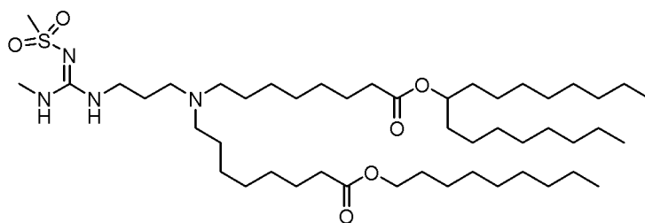
(Verbindung 212),
