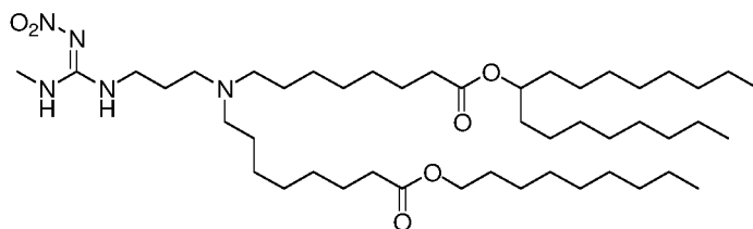
(Verbindung 200),
