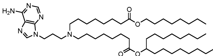
(Verbindung 45),
