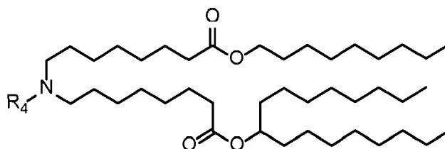
(IIa),
