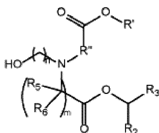
(IIId) ,
