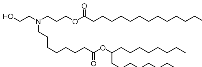
(Verbindung 97),
