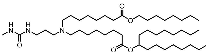
(Verbindung 41),
