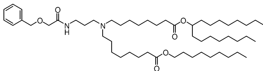
(Verbindung 197),
