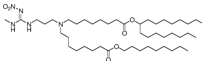
(Composé 200),
