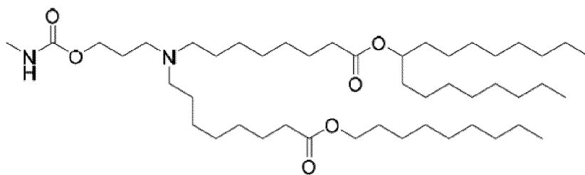
(Verbindung 175),
