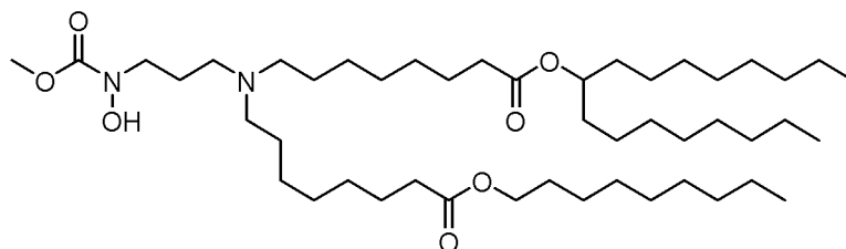
(Composé 205),
