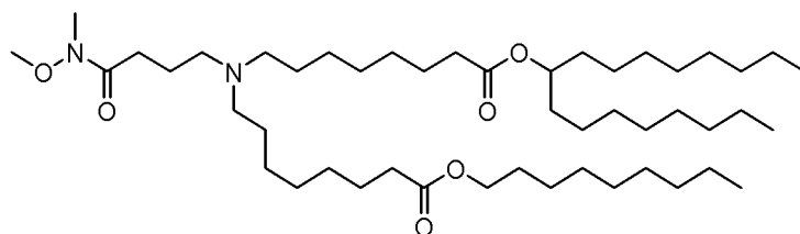
(Verbindung 228),
