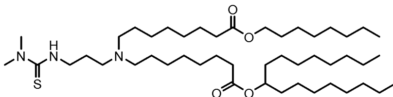
(Verbindung 40),
