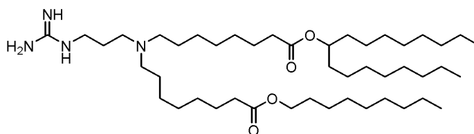
(Composé 207),
