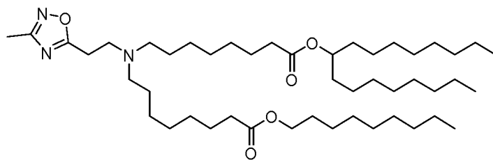
(Verbindung 230),
