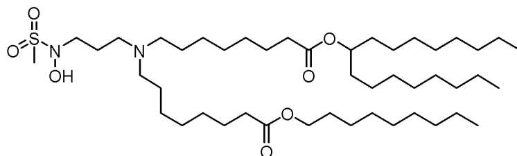
(Verbindung 206),
