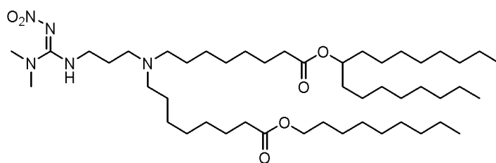
(Verbindung 209),
