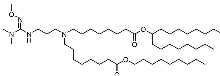
(Composé 211),
