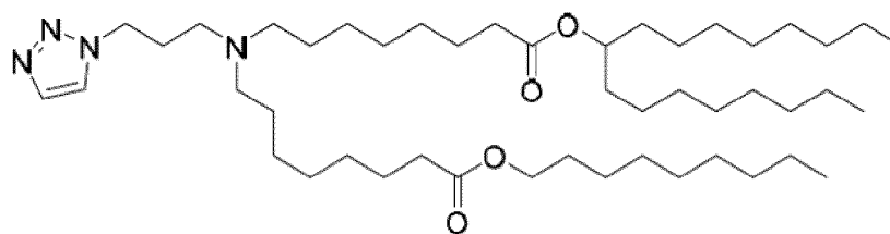
(Verbindung 179),
