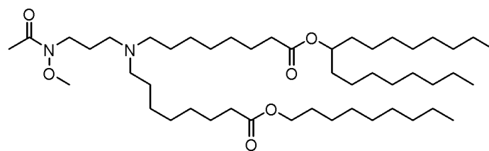
(Composé 203),
