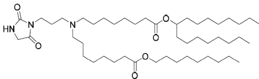
(Composé 174),
