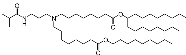
(Composé 194),
