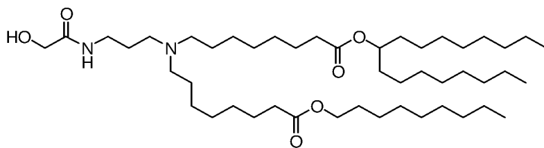
(Verbindung 198),
