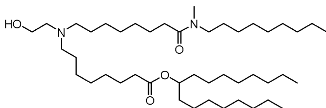
(Verbindung 105),
