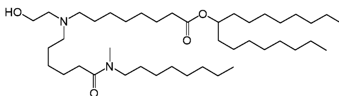
(Composé 146),
