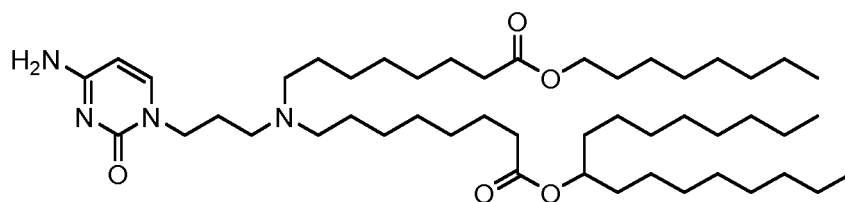
(Composé 44),
