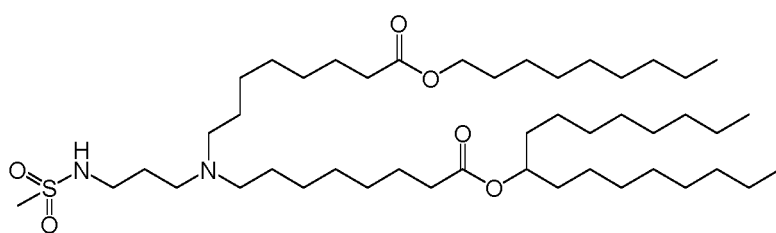
(Verbindung 109),
