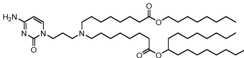
(Verbindung 44),
