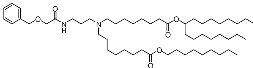
(Composé 197),
