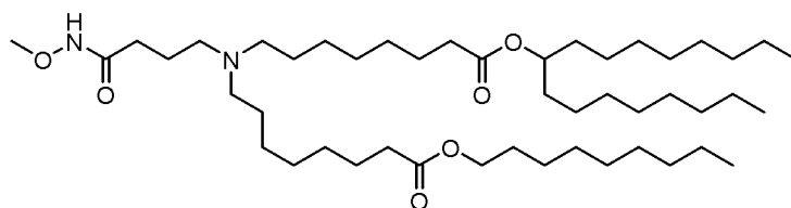
(Verbindung 226),
