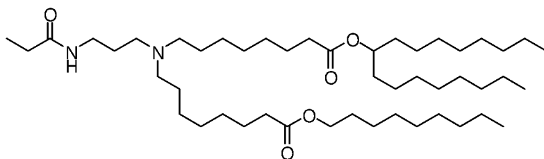
(Verbindung 193),
