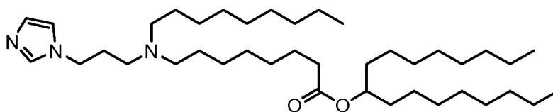
(Verbindung 8),
