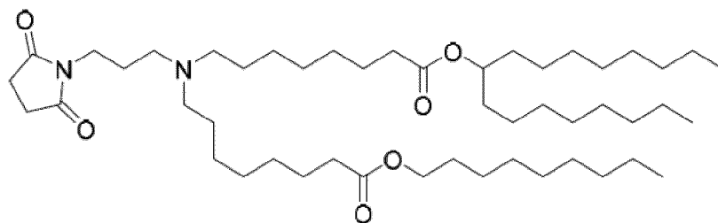
(Verbindung 176),
