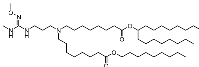
(Composé 210),
