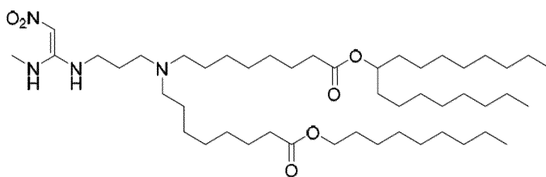
(Verbindung 170),
