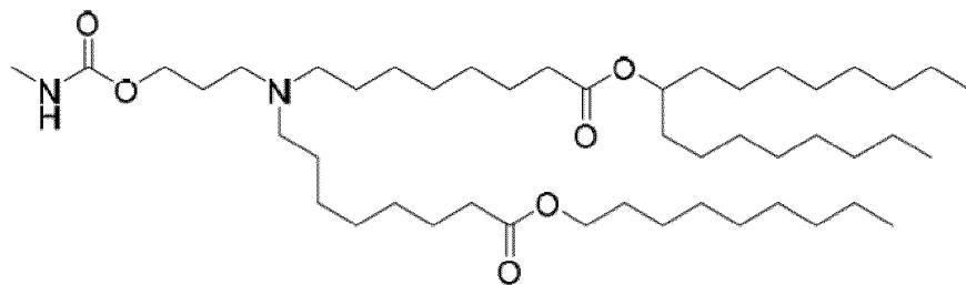
(Composé 175),
