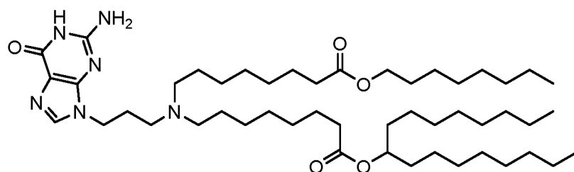
(Composé 46),
