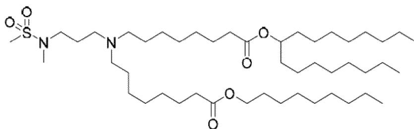
(Verbindung 173),
