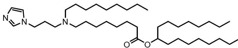
(Composé 8),
