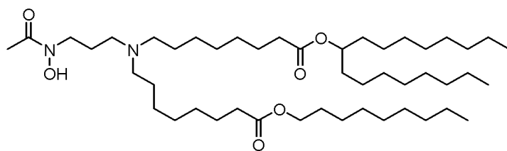
(Verbindung 204),
