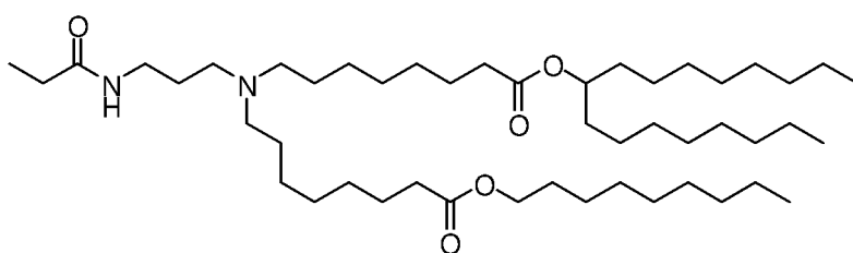
(Composé 193),
