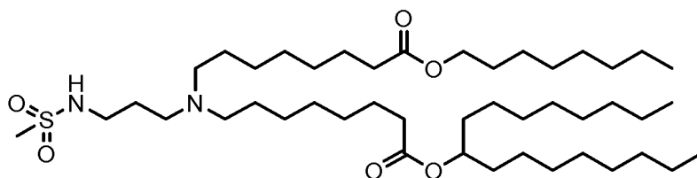
(Composé 38),
