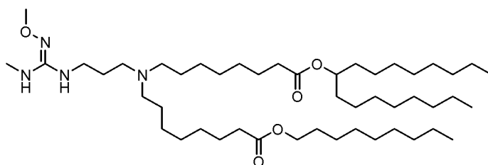
(Verbindung 210),
