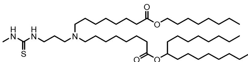
(Verbindung 42),
