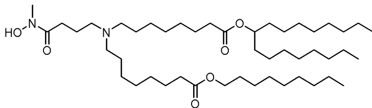
(Verbindung 227),
