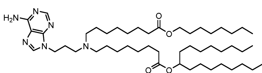
(Composé 45),
