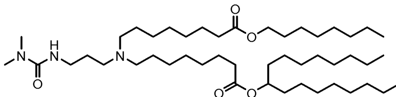
(Composé 39),
