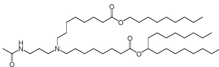
(Composé 108),
