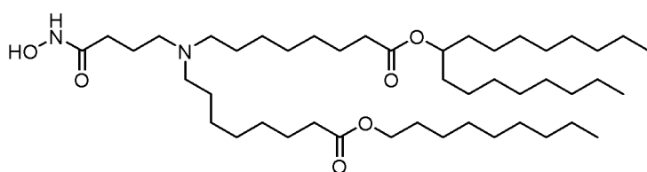
(Verbindung 225),
