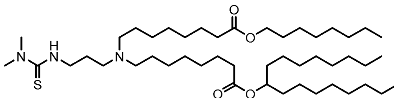
(Composé 40),
