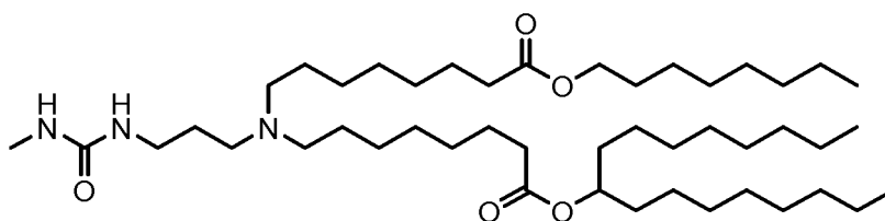
(Composé 41),
