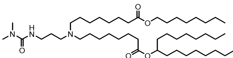
(Verbindung 39),
