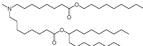
(Composé 123),
