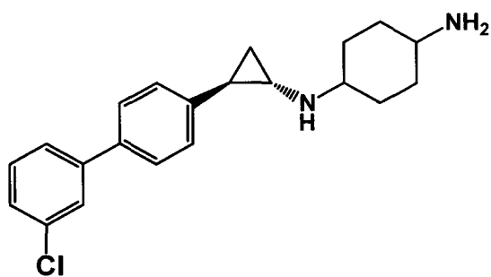
Example 62: 4'-((trans)-2-((4-aminocyclohexyl)amino)cyclopropyl)-[1,1'-biphenyl]-3-ol
