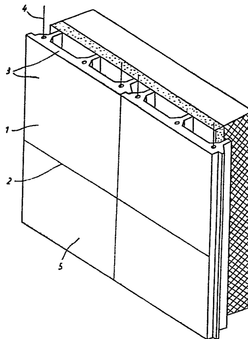
A / Fassadenvorhang für Hängefassaden
