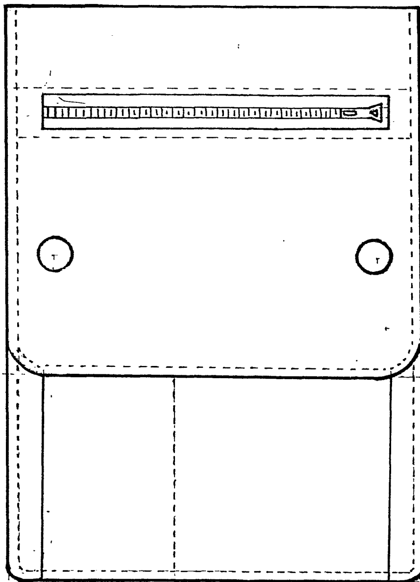
FIG. 1 VUE DE FACE FERME
