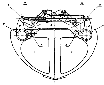
Coupe B-B
