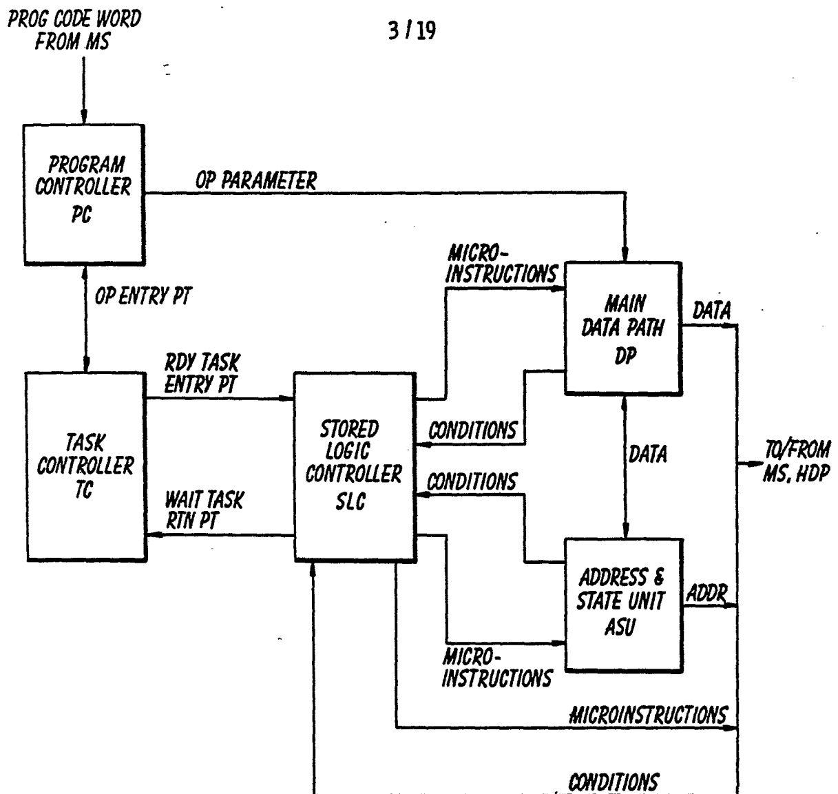
FIG. 3 PROCESSING ELEMENT PE
