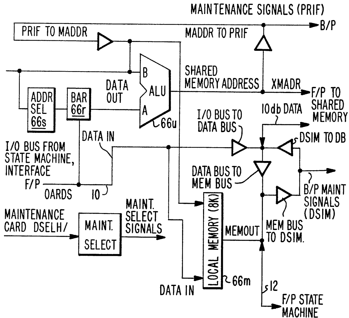
FIG. 11. MEMCTL BLOCK DIAGRAM.
