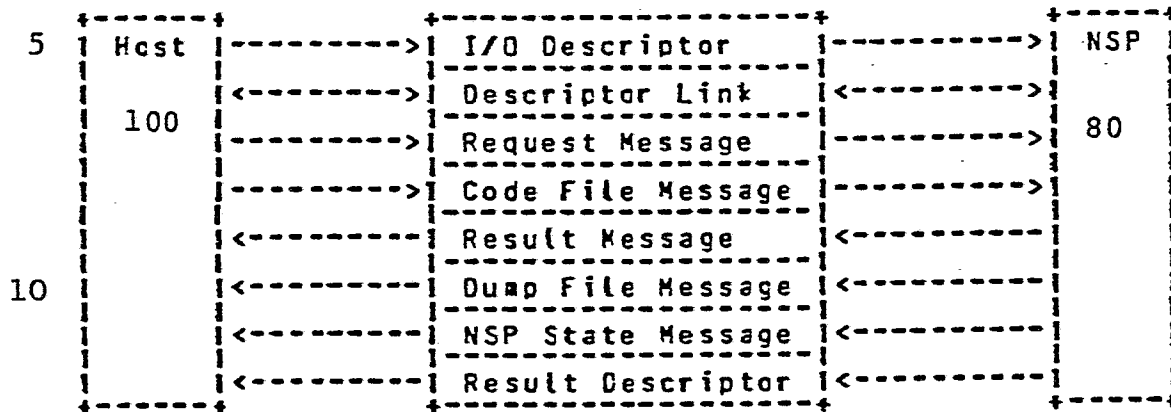
Message Types
