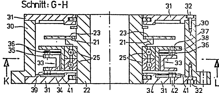
FIG. 4 Schnitt: G-H
