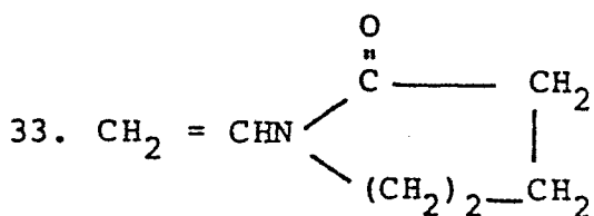
vinylvalerolactam
