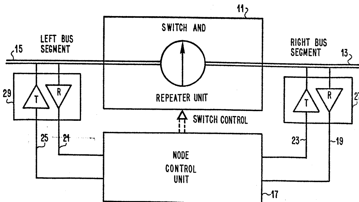
FIG. 2 NODE
