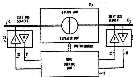
FIG. 2 NODE
