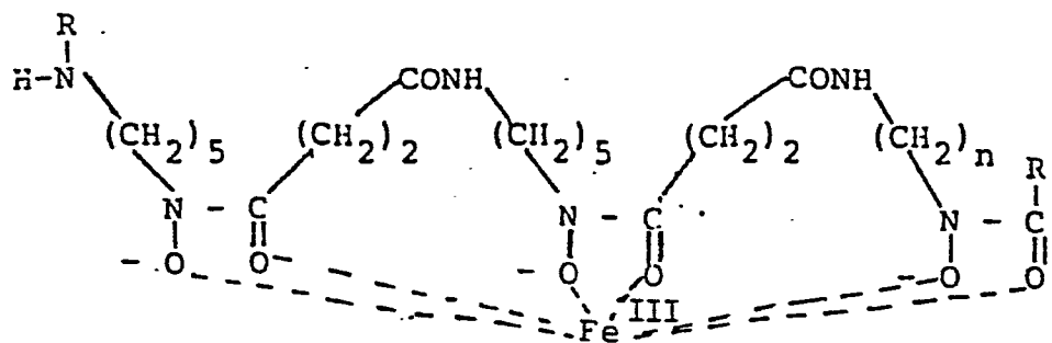
Linear ferrioxamine
