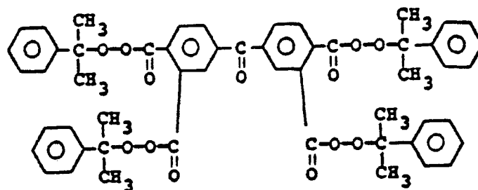
3,3',4,4'-Tetra-(p-isopropylcumylperoxycarbonyl)-benzophenone
