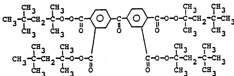
3,3',4,4'-Tetra-(cumylperoxycarbonyl)-benzophenone
