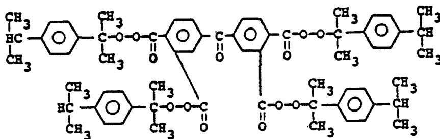
3,3',4,4'-Tetra-(p-isopropylcumylperoxycarbonyl)-benzophenone
