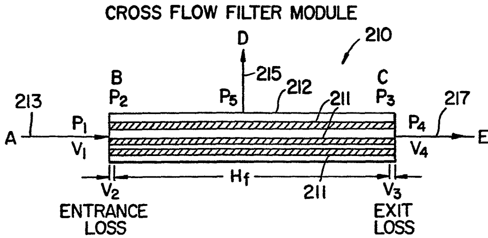
FIG. 15. 16/17 PRIOR ART
