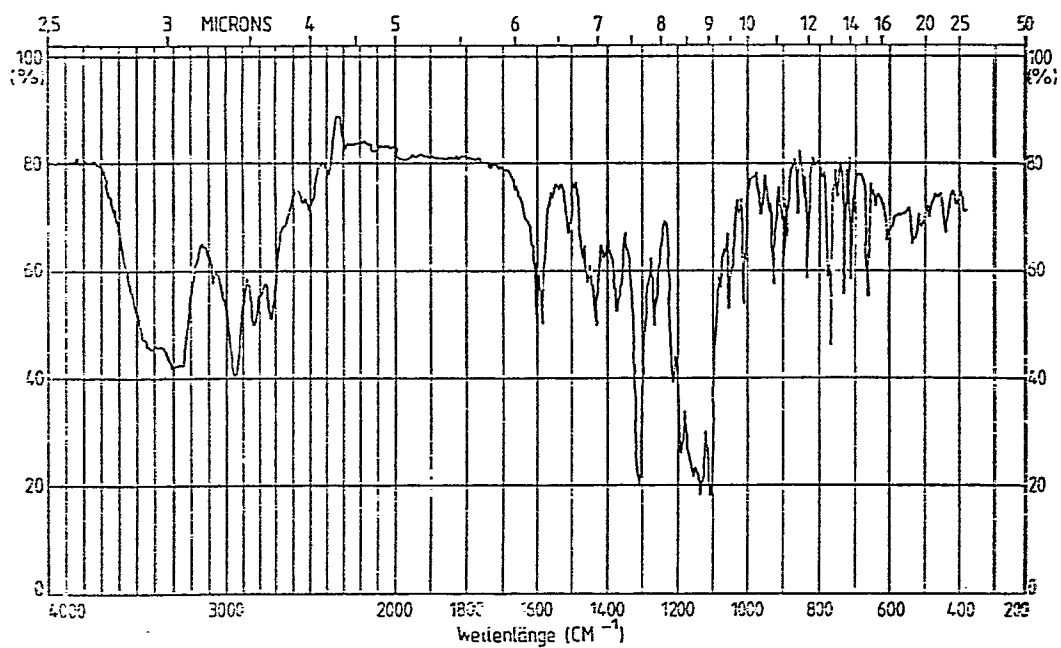
Fig. 5: Mefloquin-hydrochlorid, Modifikation E
