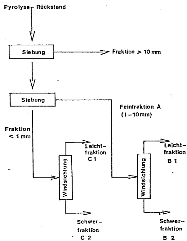
Bild 2: Fließschema der Abtrennung der kohlenstoffärmeren, mineralstoffreicheren Fraktionen über Siebung und Windsichtung
