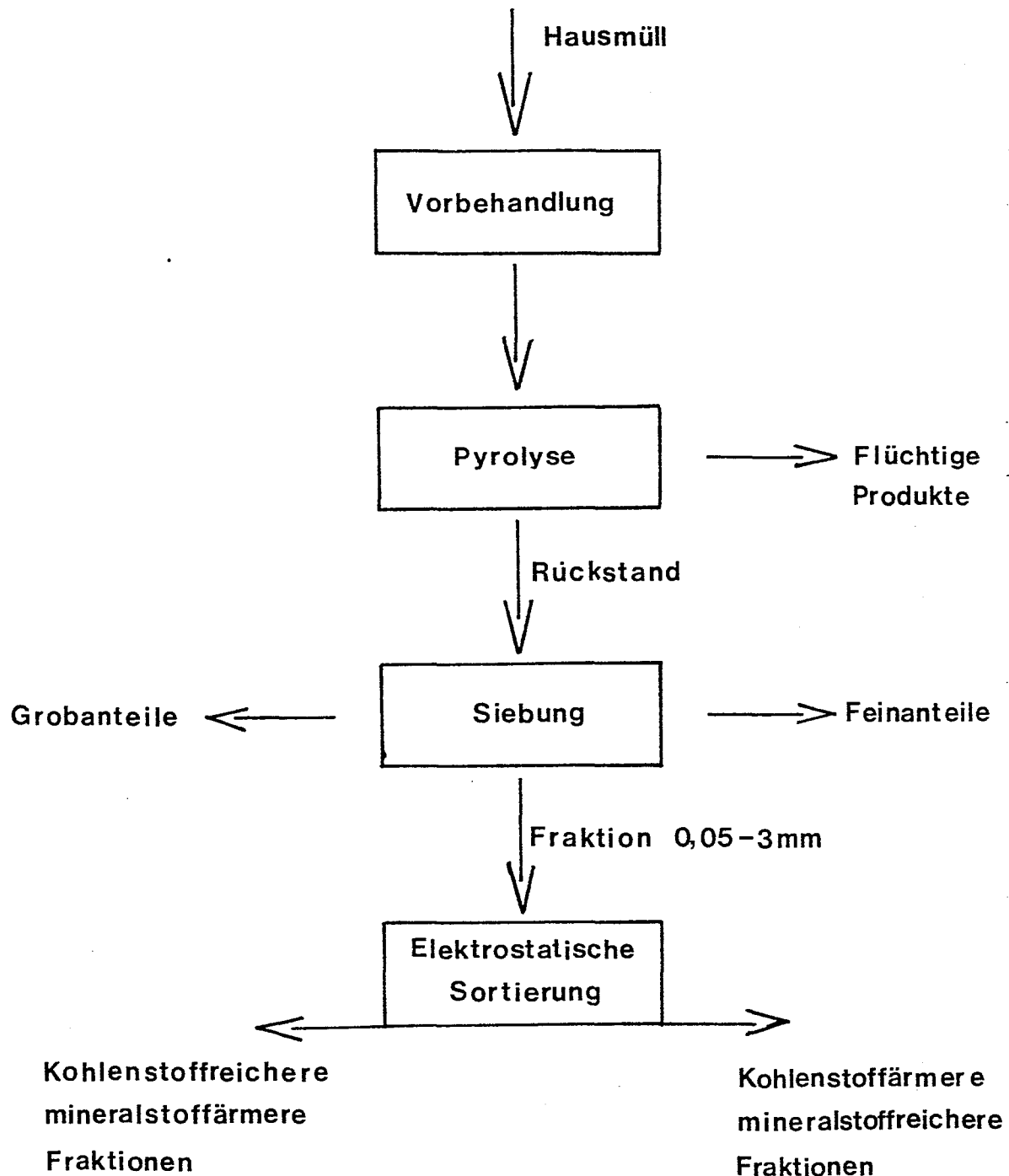
Bild 1: Fließschema der Abtrennung der kohlenstoffärmeren mineralstoffreicheren Fraktionen über elektrostatische Sortierung
