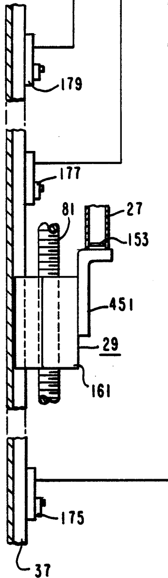
FIG. 12
