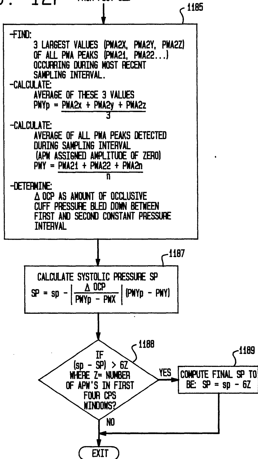
FIG. 12F FROM FIG. 12E
