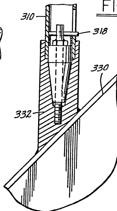
FIG. 49
