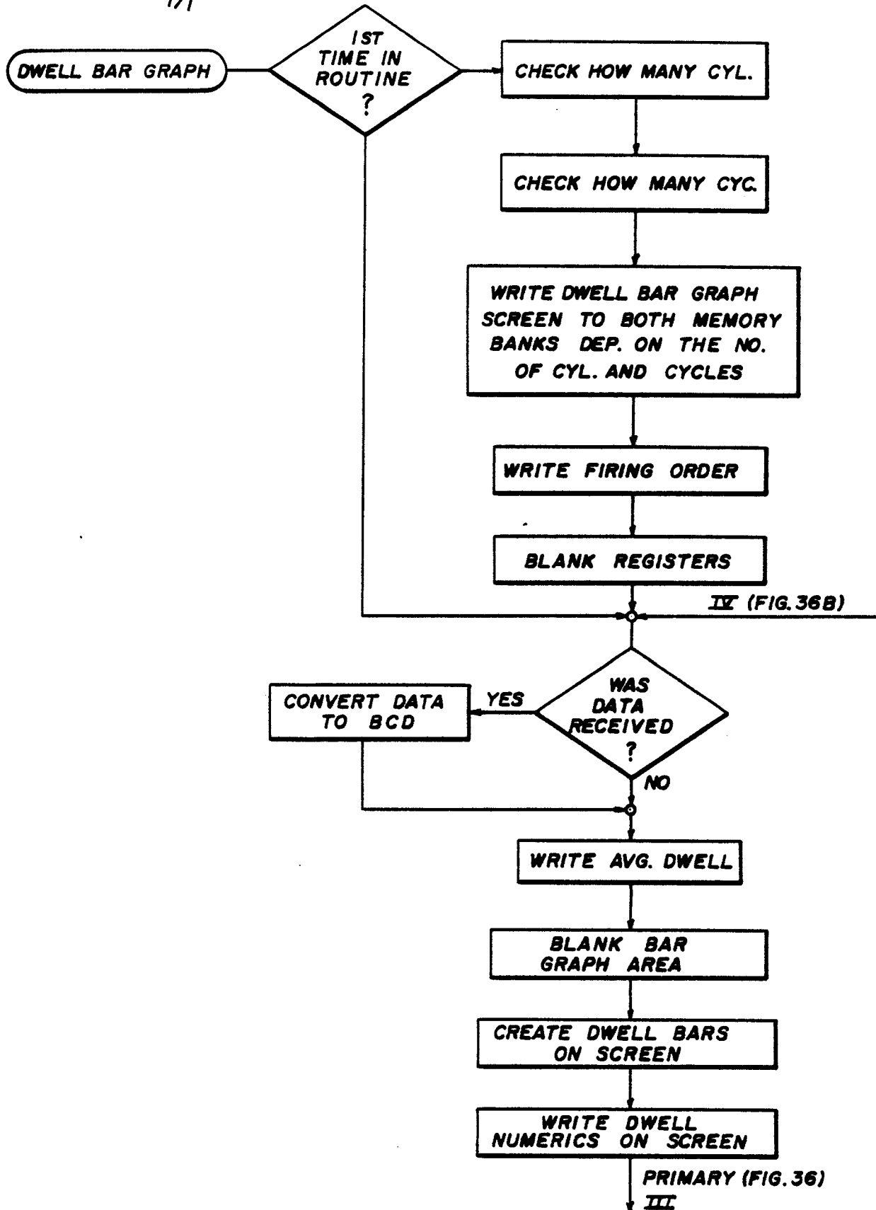
FIG.39 DWELL BAR (DISPLAY) 1/1
