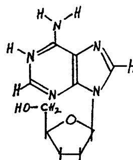
ddA
