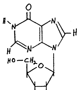
ddI
