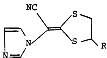
(Z isomer)
