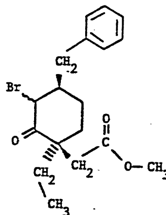
(IVb-( \pm ) cis )
