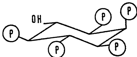
L-myo-inositol-1.2.3.4.5-penta- phosphate or L-1.2.3.4.5-IP 5
