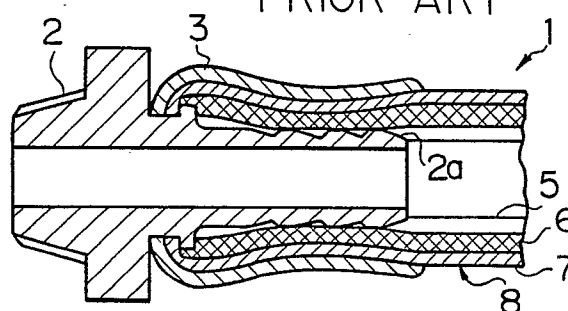
FIG. 15 PRIOR-ART
