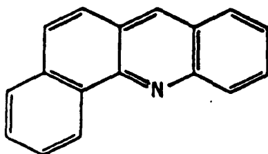
Benz[c]acridine
