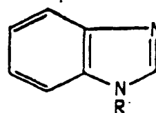
Benzimidazole
