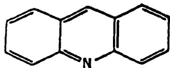
Acridine
