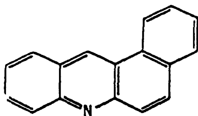
Benz[a]acridine
