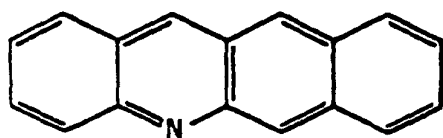
Benz[b]acridine
