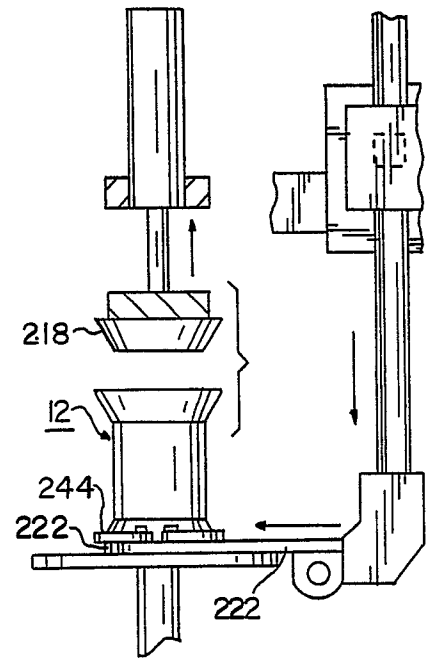
FIG. 5C
