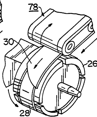
FIG. 6E
