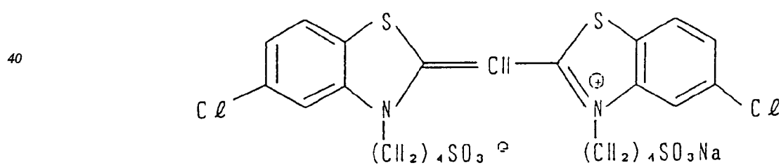
E x S - 6
