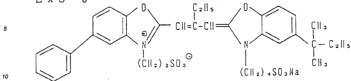
E x S - 3
