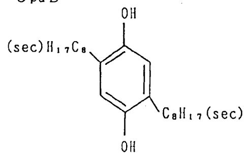
C pd B
