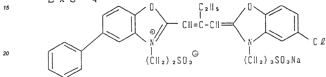
E x S - 4
