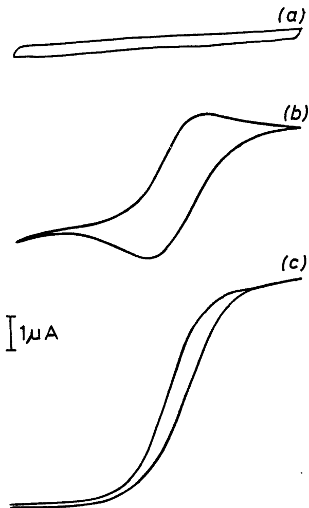
FIG.12. 0 +200 +400 E/mV vs.SCE.
