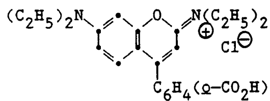
Rhodamine B
