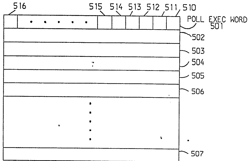
FIG. 5 POLLING TABLE
