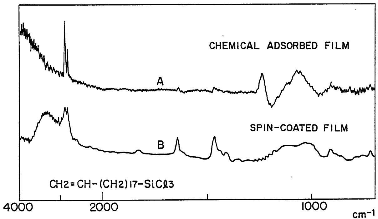
FTIR SPECTRUM
